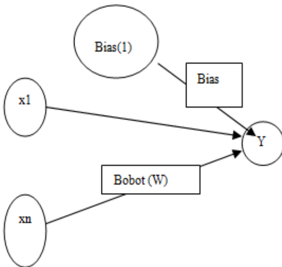
Gambar.2 . Arsitektur perceptron lapis tunggal
