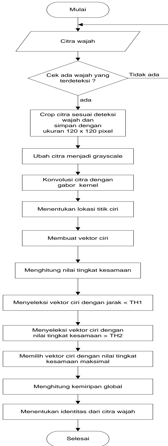
Gambar 6. Flowchart Pengidentifikasian Wajah
