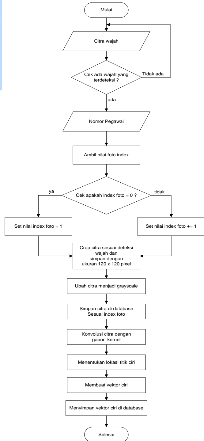
Gambar 5. Diagram Alir Pengambilan Citra Referensi
